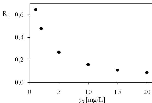
Figure 9. Values of separation factor R_L for sorption of ENRO by natural zeolite Slika 9. Vrijednosti faktora separacije, R_L za sorpciju ENRO na prirodni zeolit
